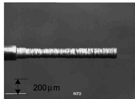
(d) Electrode machined using running wire
